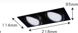
115*219mm 無邊框請準確開孔
